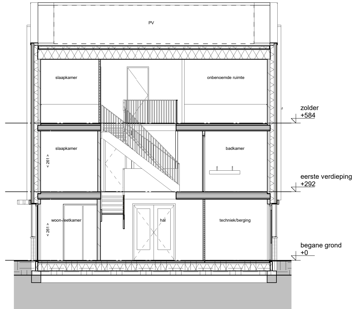
langsdoorsnede
