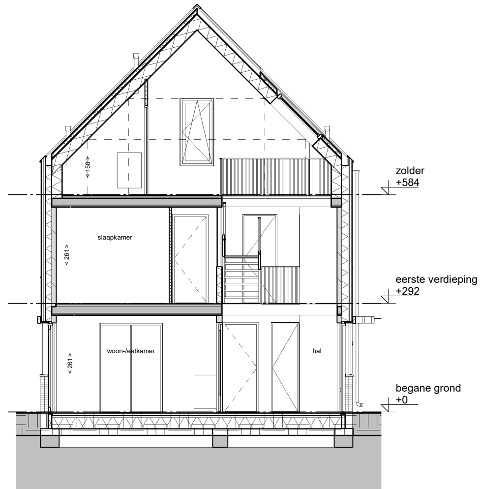
dwarsdoorsnede
